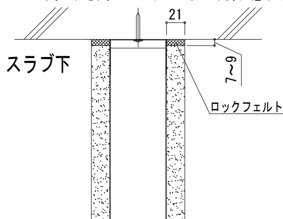
<スラブ下の納まり例>
